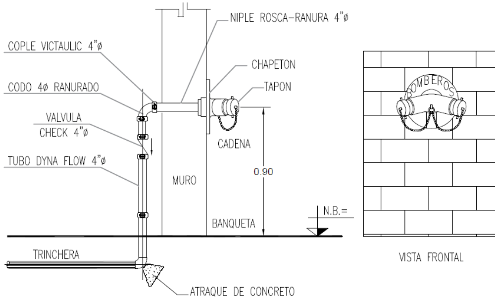
Figura 2.7- Toma siamesa.
