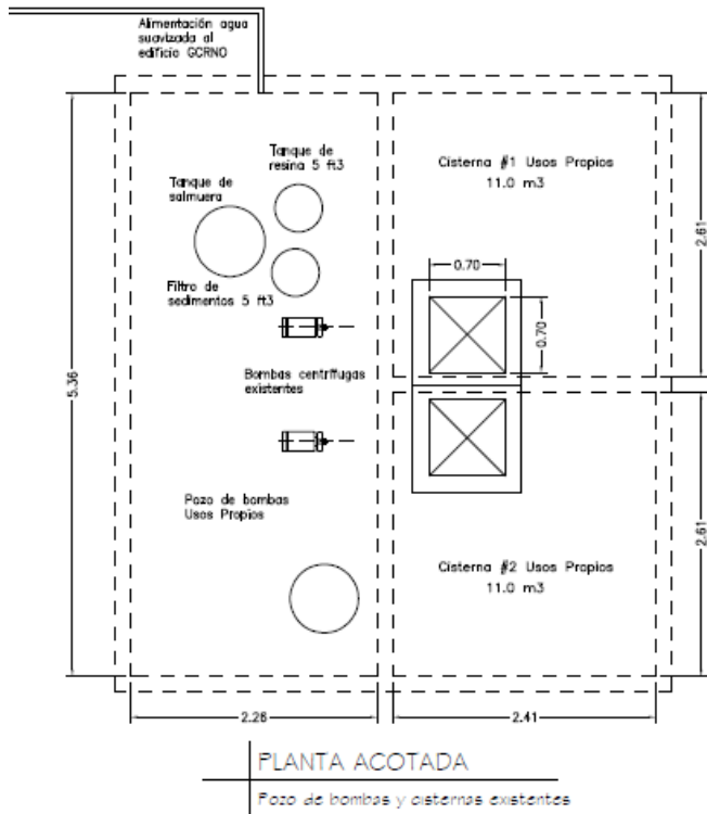
Figura 1.2- Disposición existente de pozo de bombas.
